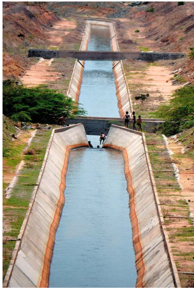
ໝອງຝາຍນໍ້າຮອງຂອງໂຄງການລະບາຍນໍ້າໄຊເກີດ-ເຊສະລະລອງແຂວງສະຫວັນນະເຂດເຊິ່ງແມ່ນກຸ່ມບໍລິສັດຫຸ້ນສ່ວນເກີໂຈວບາຈີນເປັນຜູ້ຮັບເໝົາກໍ່ສ້າງ 由中国葛洲坝集团股份有限公司承建的老挝沙湾拿吉省色萨拉龙—赛格灌溉项目引水干渠
